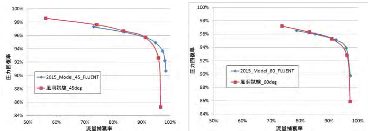
図5 風洞試験結果とCFD解析の比較 左： 45^\circ モデル 右： 60^\circ モデル
