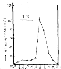
第25圖 示差曲線 (Pt + -Ag)
