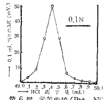
第6図 示差曲線 (Pt + -Ni)
