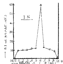
第41图 示差曲线 (Pt + -W)
