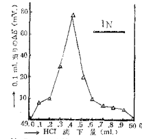
第5図 示差曲線 (Pt + -Ni)
