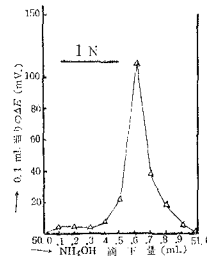
第9図 示差曲線 (Pt + -Ni)
