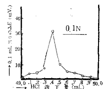
第22圖 示差曲線 (Pt + -Ag)
