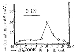
第50図 示差曲線 (Pt + -W)
