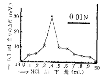
第7図 示差曲線 (Pt + -Ni)
