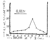
第11図 示差曲線 (Pt + -Ni)
