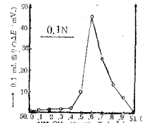
第10図 示差曲線 (Pt + -Ni)
