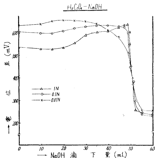
Fig. 2. Pt + -Ni 滴定曲線
