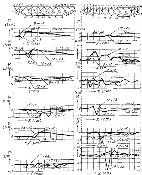
第7図 材端モーメント(M)影響線 (4)
