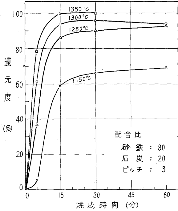
図-3 還元度におよぼす焼成時間の影響
