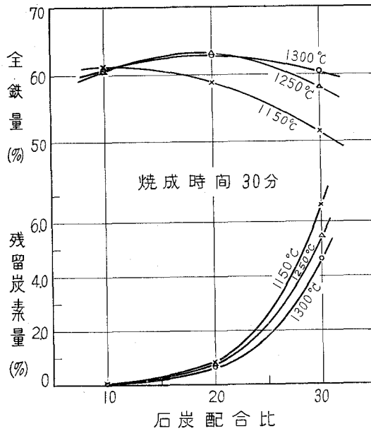
図-7 全鉄および残留炭素量におよぼす石炭配合比の影響
