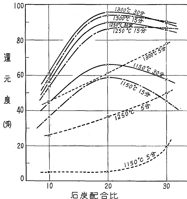
図-5 還元度におよぼす石炭配合比の影響
