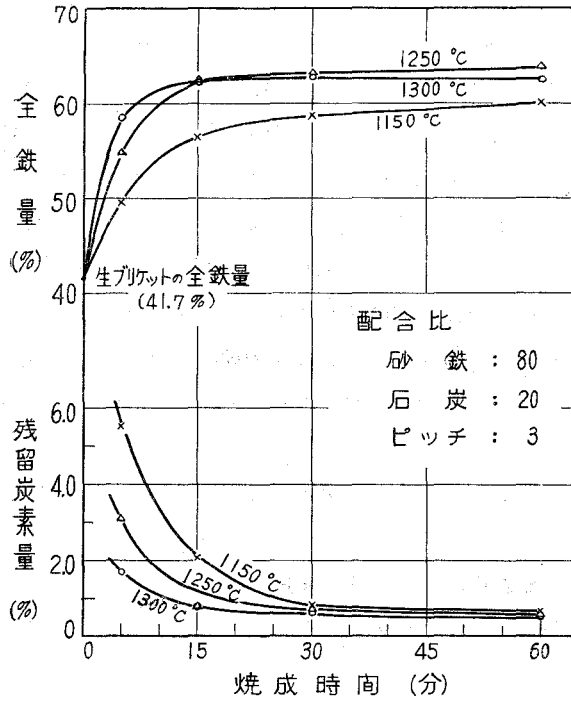
図-6 全鉄および残留炭素量におよぼす焼成条件の影響
