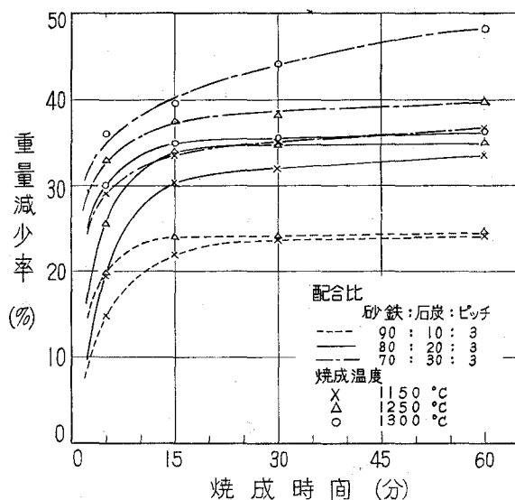
図-2 焼成ブリケットの重量減少率
