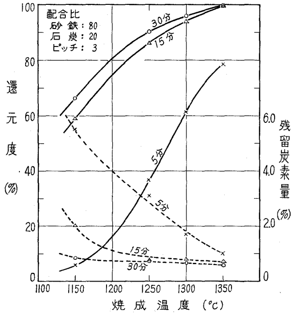
図-4 還元度および残留炭素量におよぼす焼成温度の影響
