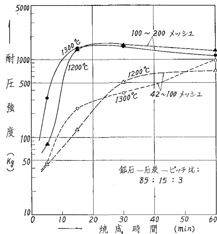
図-8 耐圧強度におよぼす鉄石粒度の影響
