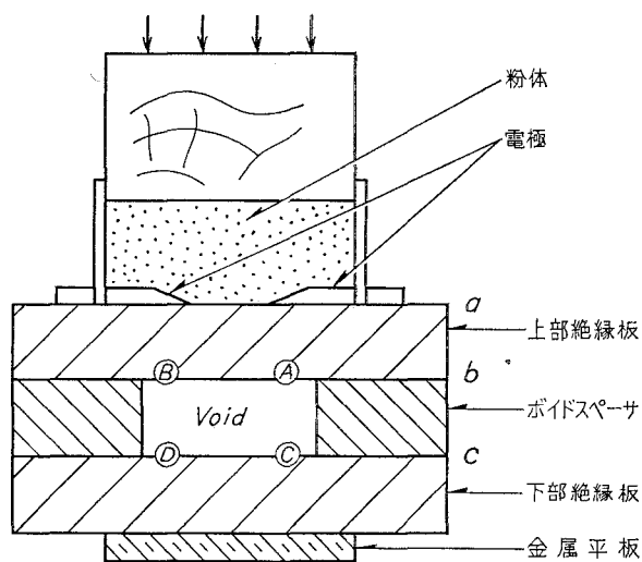
図-1 実験装置
