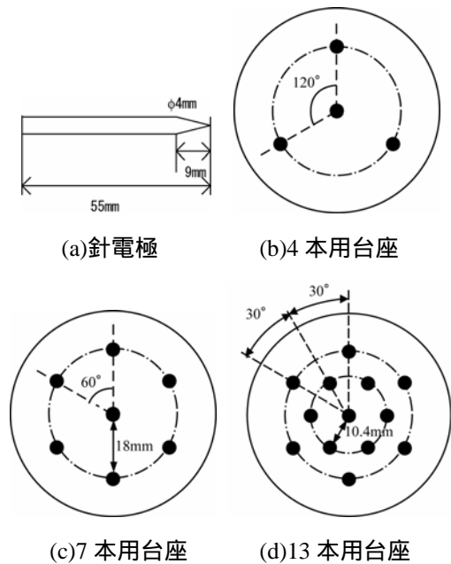
図 2 針電極と台座
