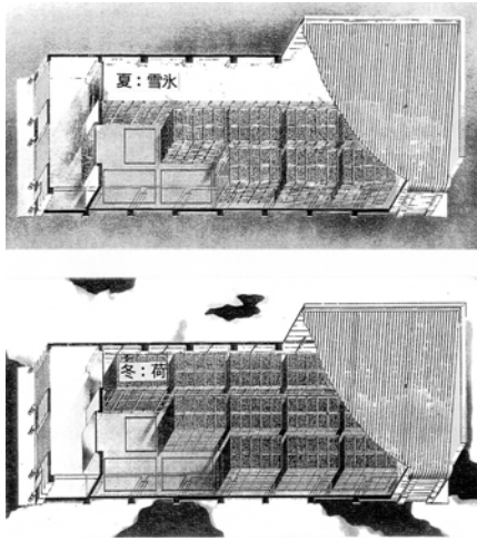
図2 水室型農産物長期保冷庫
