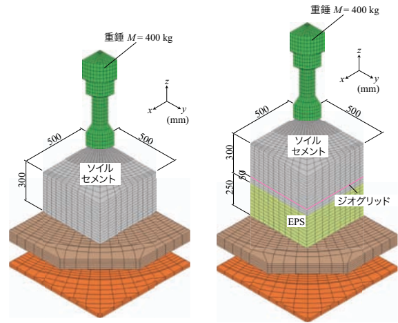
(a) ソイルセメント単体の場合 (b) ジオグリッド埋設ソイルセメントと EPS の場合
