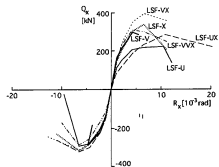
図-7 x方向荷重-変形包絡線
