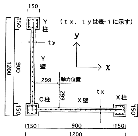
図-2 壁断面
