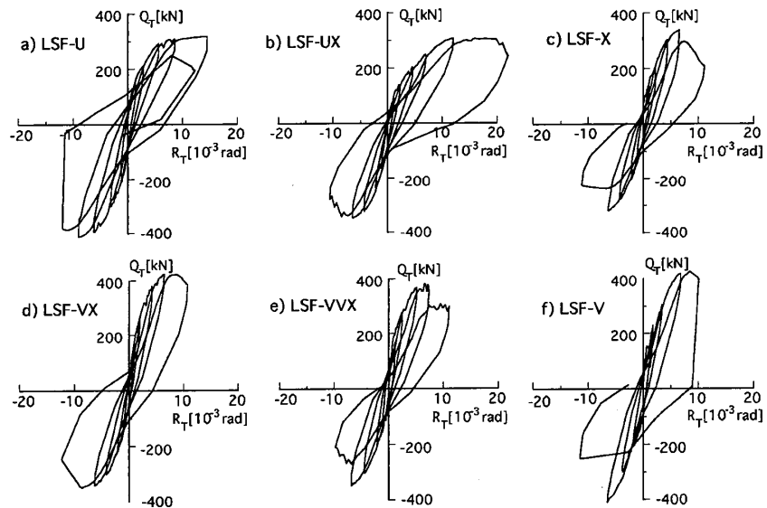
図-6 荷重方向荷重-変形曲線
