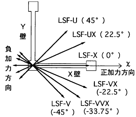
図-4 荷重方向と試験体名
