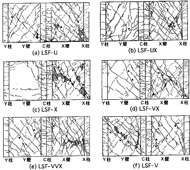
図-5 ひび割れおよび破壊状況
