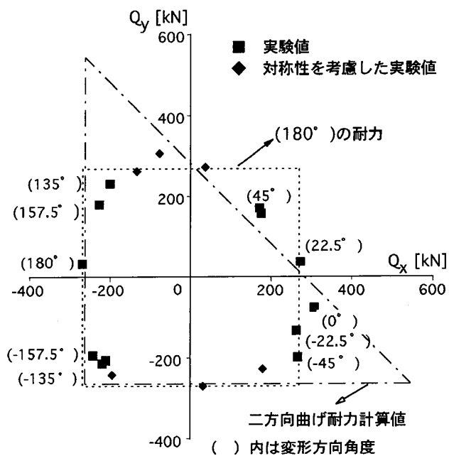
(b) 変形方向を定めた実験[4]
