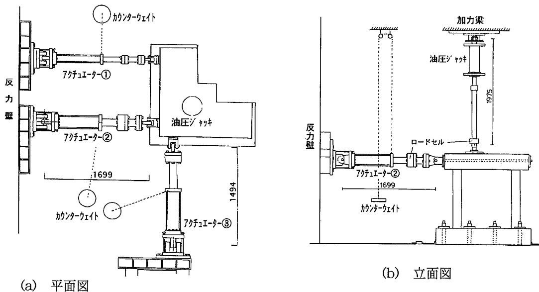
図-3 加力装置概要 単位 (mm)
