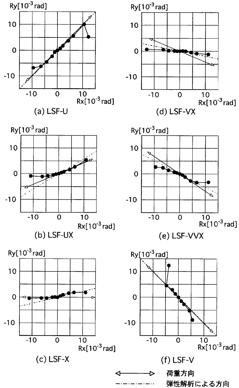
図-8 荷重方向と変形方向
