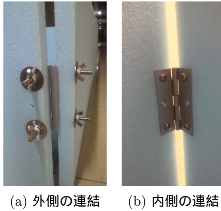
図 5.17: スタイロフォーム IB を使用した壁とその連結
