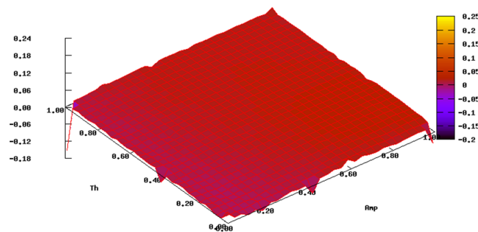
図 3.35: 提案システムと \epsilon -greedy 法 + 加重平均手法との平均獲得報酬の差
