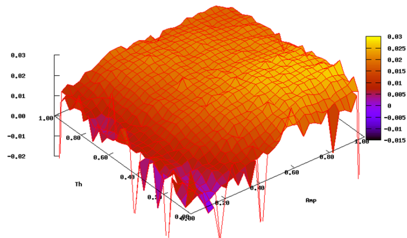
図 3.38: 提案システムと \epsilon -greedy 法 + Q 学習の平均獲得報酬の差 (拡大)
