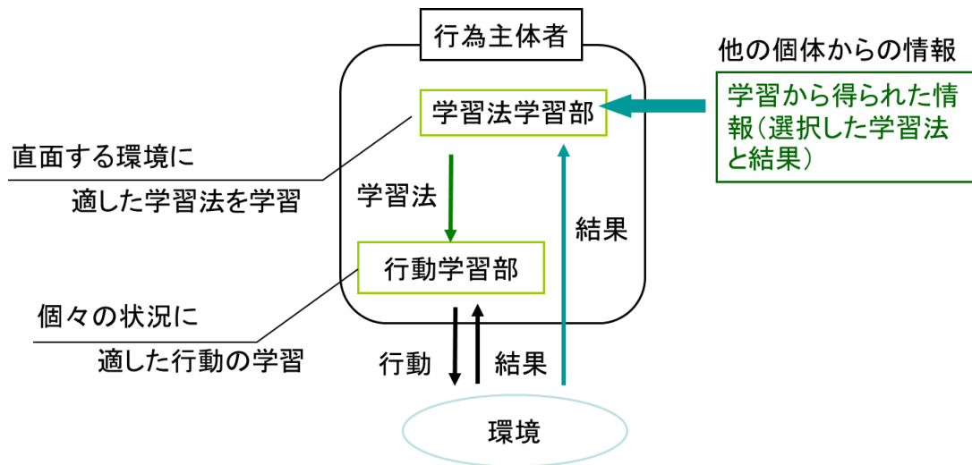
図 3.5: 学習法をコミュニケーション情報とした個体学習促進システムの概念図
