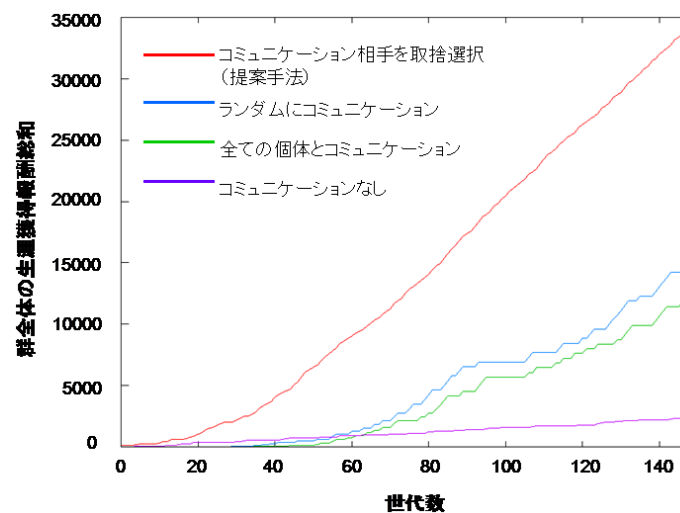
図 4.18: 群全体の獲得報酬総和
