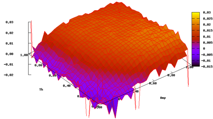
図 3.31: 提案システムと softmax 法 + 加重平均手法の平均獲得報酬の差 (拡大)
