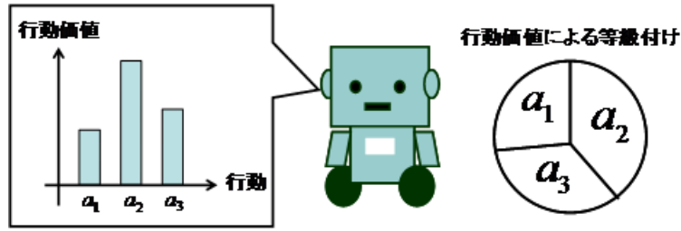
図 2.6: softmax 法
