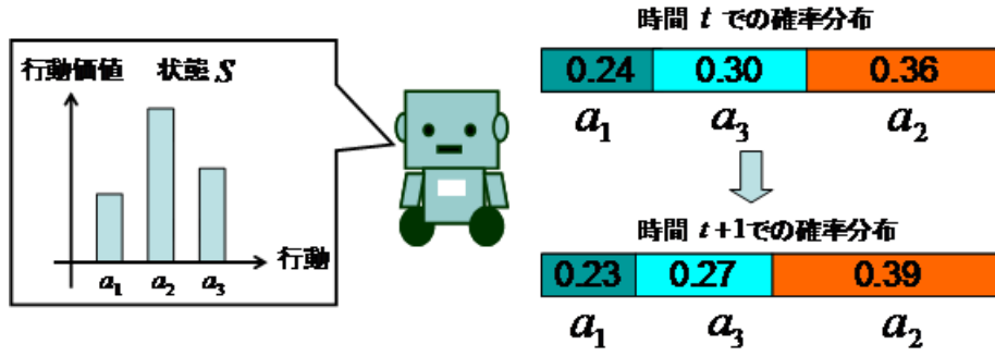
図 2.7: 追跡手法
