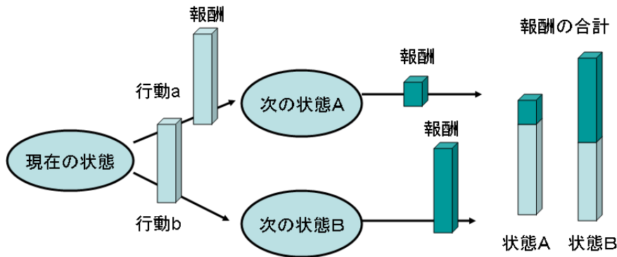
図 2.8: Q 学習法
