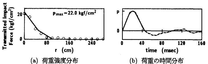
図-2 入力荷重
