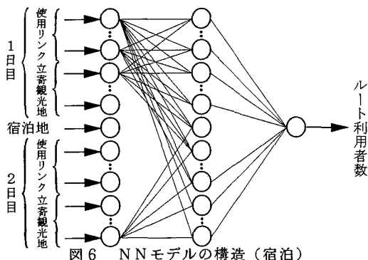
図6 NNモデルの構造（宿泊）
