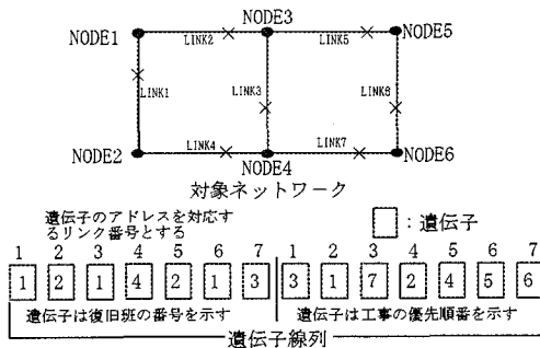
図-2 線列設計
