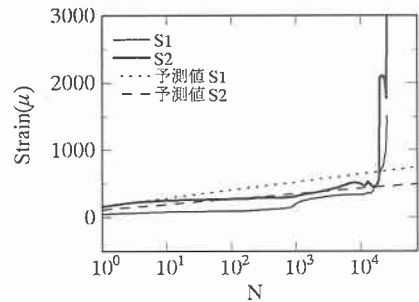
(d) No.14 V_{max}=37.1\text{kN} p_w=0.40\%
