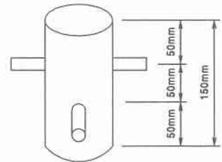
図-1 AEセンサー位置
