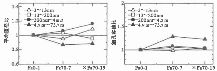
図-19 大気中疲労、上限応力比70% (周辺部)
