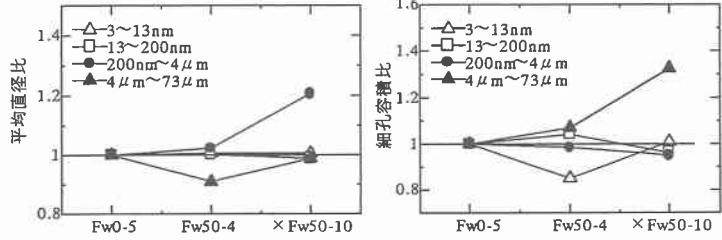
図-11 水中疲労、上限応力比50%（中心部）
