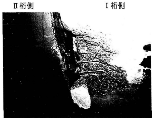
N-N-S2 の破壊状況写真
