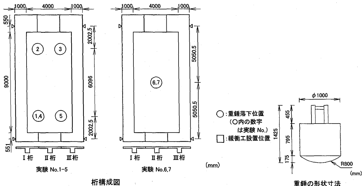
図-4 各実験ケースの桁構成および重錘の形状寸法
