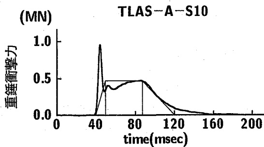
(a) 全体波形
