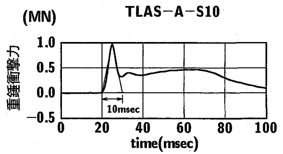
(b) 芯材衝突時の波形
