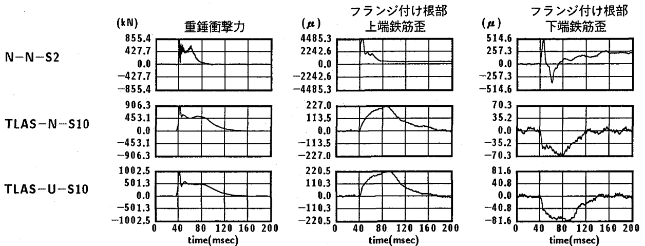
図-6 重錘衝撃力およびフランジ付け根部上下端鉄筋の歪の波形分布性状
