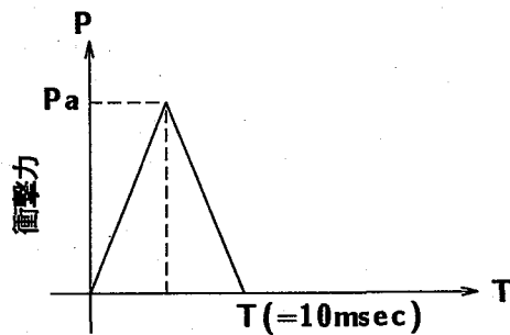
図-11 作用衝撃力波形分布
