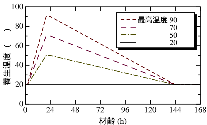
図 - 1 温度履歴
