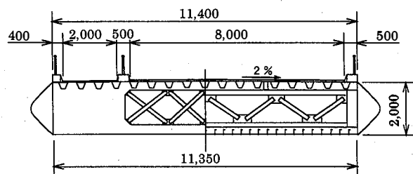
(d) 補剛桁断面図
