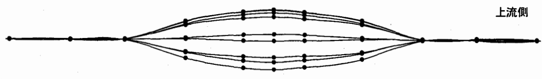
(f) ねじり一次振動 (3.15Hz)
