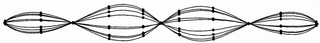
(d) 逆対称一次振動 (1.22Hz)
