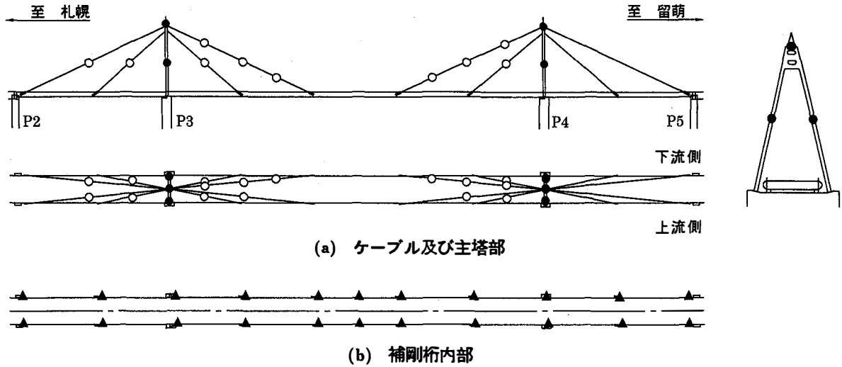
図-2 加速度計配置位置および計測振動方向成分
