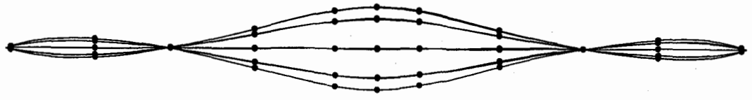
(a) 対称一次振動 (0.71Hz)
