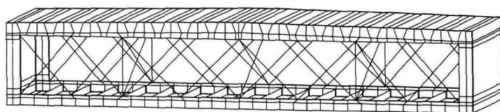
(b) 補剛桁内部
