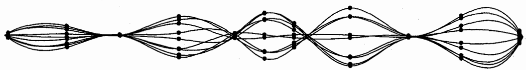
(c) 対称三次振動 (2.76Hz)
