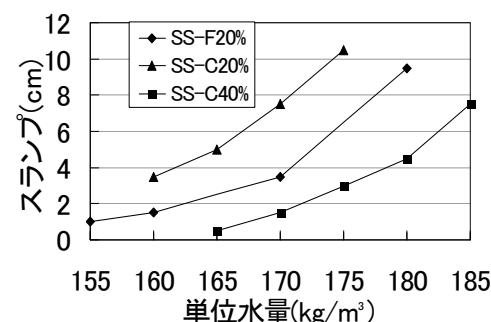
図-2 スランプ
