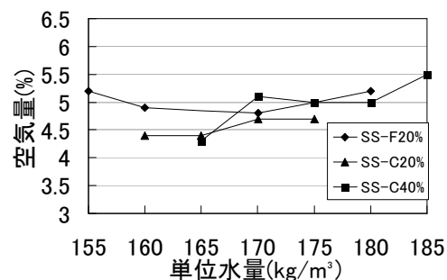
図-3 空気量
