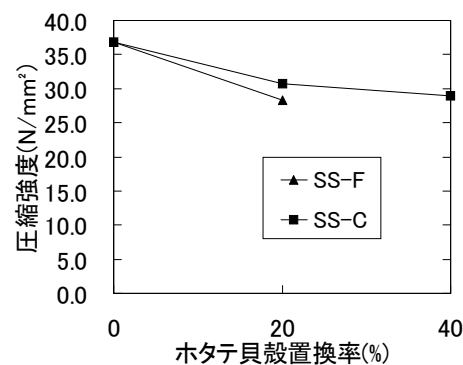
図-4 圧縮強度
