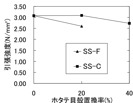
図-5 引張強度
