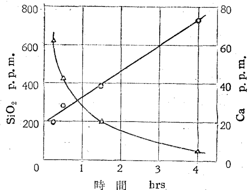
第 6 図 (\text{NaPO}_3)_6 による缶石の溶解
