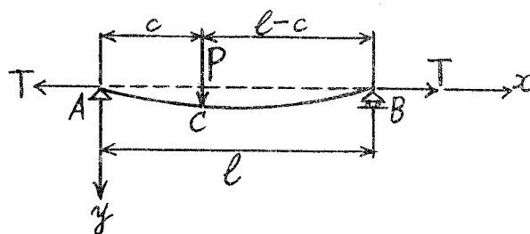
第4図 三角級数による軸力ある梁の図
