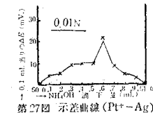
第27図 示差曲線 ( \text{Pt}^+ - \text{Ag} )
