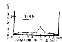
第67図 示差曲線 (Pt + —Sb)
