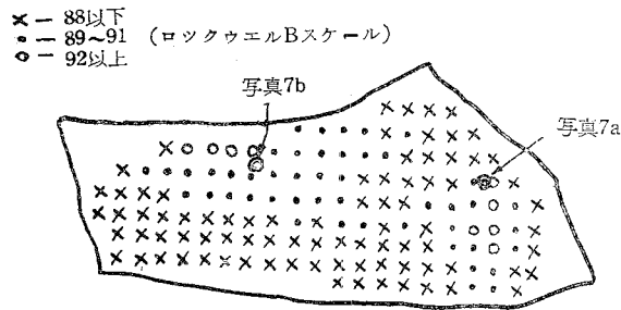
第10図 試片A-IV-I外面の硬変分布および写真7a; 7bの場所
