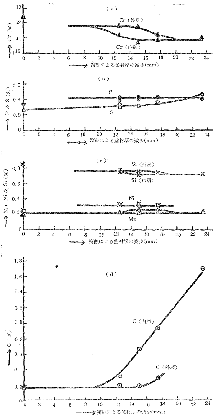
第 8 図 釜材の腐蝕による成分の変化
