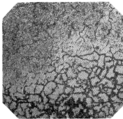
写真 6b. 6a. の拡大 \times 90 \times \frac{8}{9}
