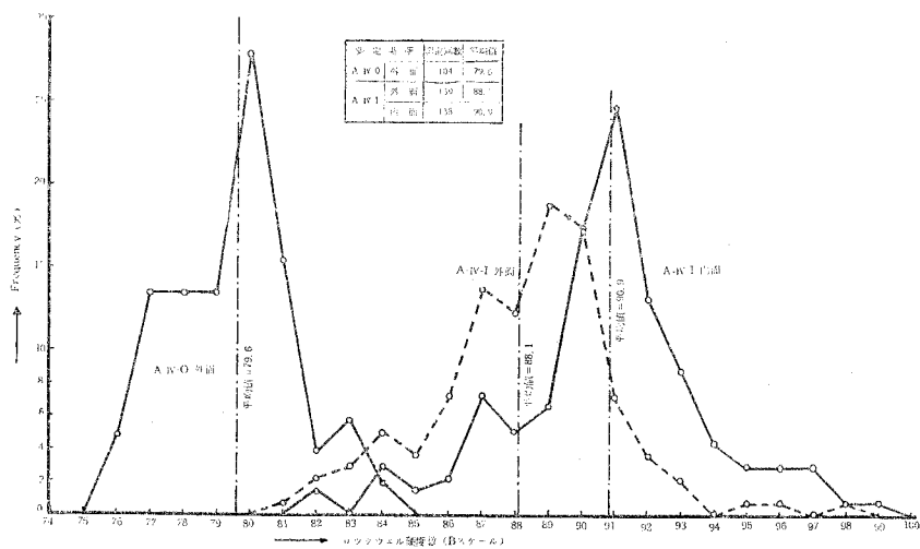
第 7 図 試片A-IVの硬度分布 (ロックウェルBスケール)
