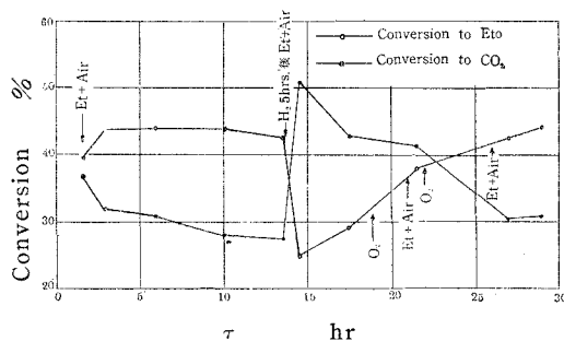
第8図 触媒の水素処理及酸素処理
