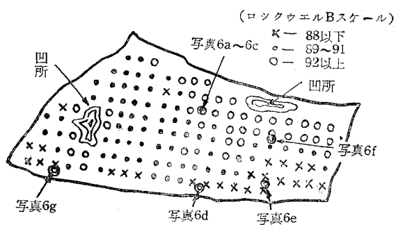
第9図 試片A-IV-1内面の硬度分布 および写真5a~6gの場所
