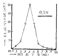
第6図 示差曲線 (Pt + -Ni)
