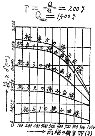
第15圖 孟宗竹梁の荷重点撓度 W - d 曲線
