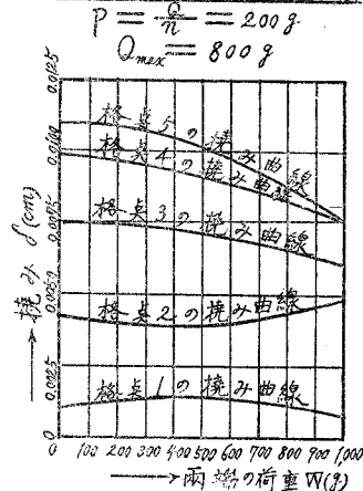
第16圖 鋼鉄梁の荷重点撓度 W - d 曲線
