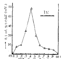
第5図 示差曲線 (Pt + -Ni)
