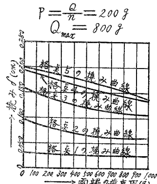
第16圖 鋼鉄梁の荷重点撓度 W - d 曲線
