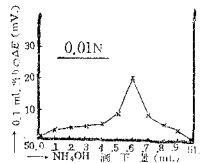
第11図 示差曲線 (Pt + -Ni)
