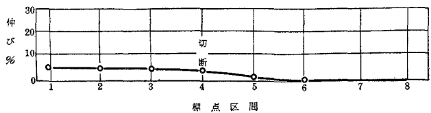
第6図 試験片 No. 4 (-183°C)
