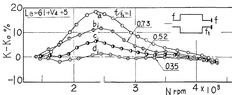
図-20 (K - K_0) 曲線 ( f/f_e 変化)
