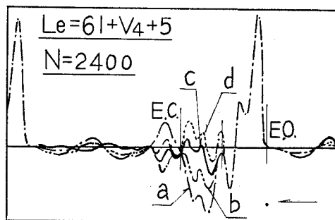
図-21 オシログラム ( f/f_e 変化)
