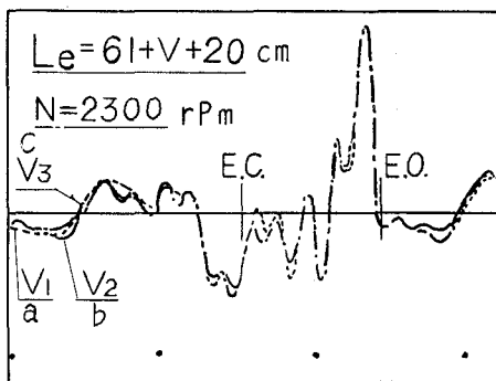
図-4 オシログラム ( V 変化)
