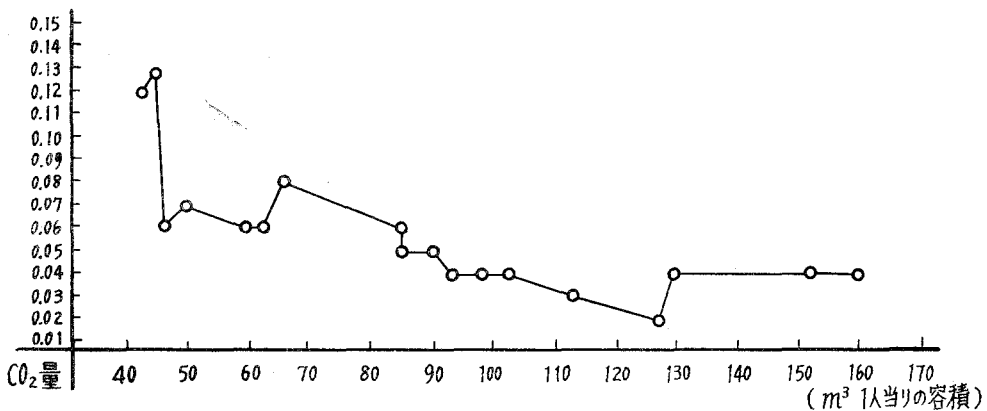
図-13 運動中のCO 2 の量と気積
