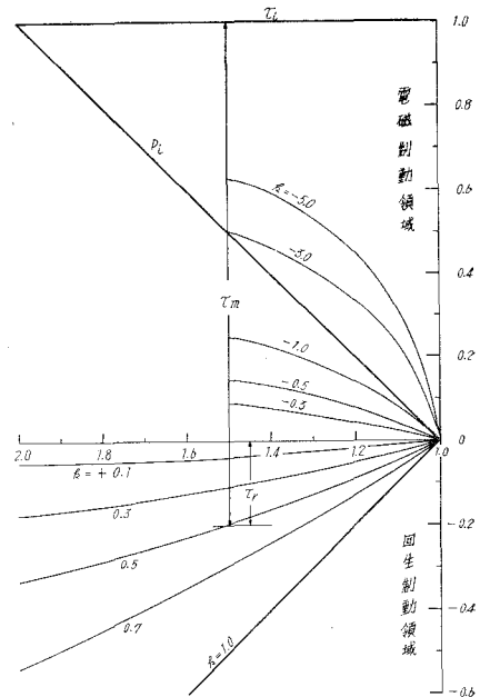
図-10 出力，トルク特性 ( s > 1, k < 0; s > 1, k > 0 )
