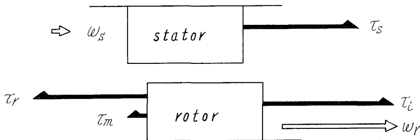
図-4 トルク配分 ( s < 0 , k < 0 )
