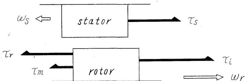
図-1 トルク配分 ( 0 < s < 1, k > 0 )
