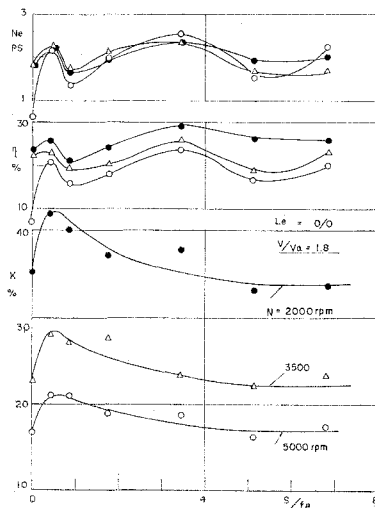
図-23 入口面積と機関性能 ( L_e=0/0 , V/V_h=1.8 )
