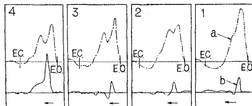
図—13 排気絞り弁の位置と給気比 (E-50, C-4/4)
