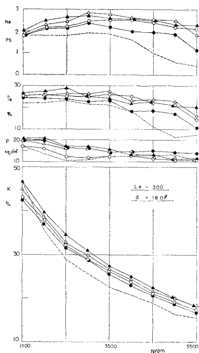
図-16 排気絞り弁位置と機関性能 ( L_e=200 , d=18.0\phi )
