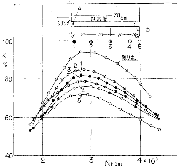
図—12 開口端絞り弁と給気比、機関トルクの増加 (E-50, C-4/4)
