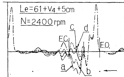
図-10 オシログラム ( f/f_0 変化)
