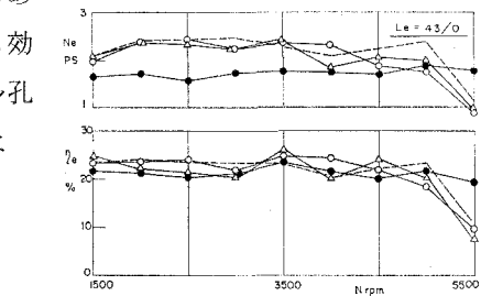
図-22 多孔共鳴型消音器の容積 と機関性能 ( L_e=43/0 , s/f_e=2.57 )
