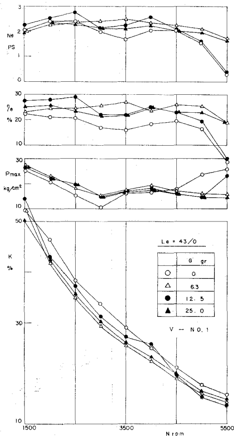
図-31 グラス・ウール充填量の効果 ( Le=43/0 , V-No. 1)
