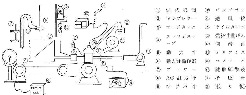
図-1 実験装置
