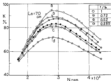
図-4 排気絞り弁面積と給気比 (C-4/4, E-50)
