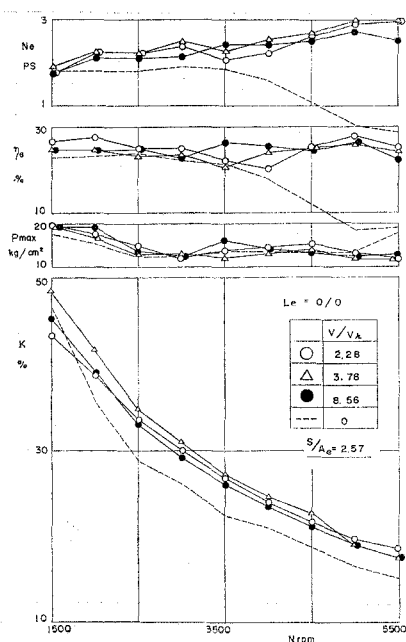
図-20 多孔共鳴型消音器の容積と機関性能 ( L_e = 0/0 , s/A = 2.57 )
