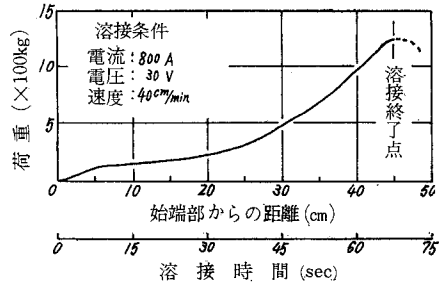
図-7 荷重曲線
