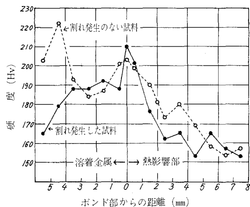
図-9 終端部試料の硬度
