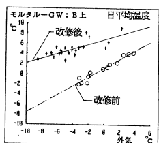
図-55 外気-B壁内温度(上)
