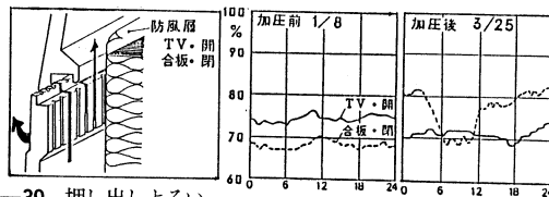
図-40 壁内湿度
