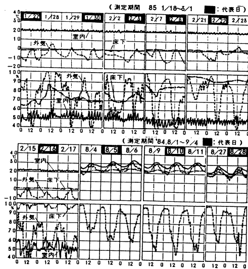
図-11 室内外温湿度状況
