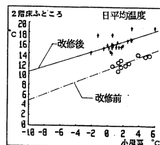
図-54 小屋裏-2階床ふとところ
