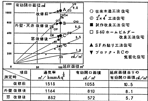
図-48 住宅の気密性能測定結果
