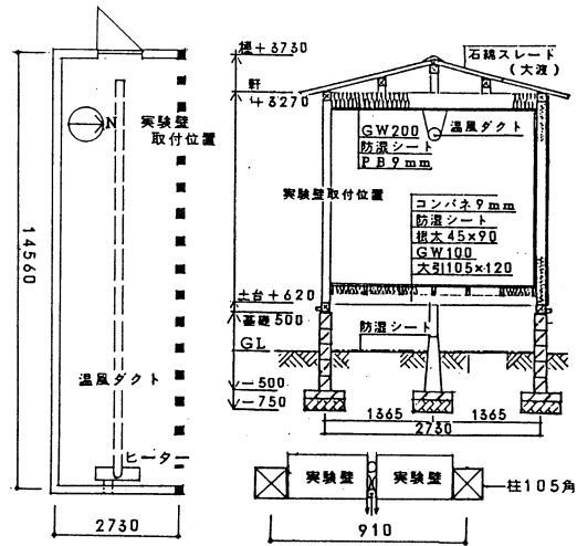
図-10 実験棟の概要
