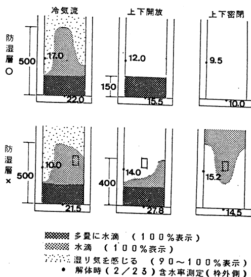
図-17 サイディング壁下部の結露状況
