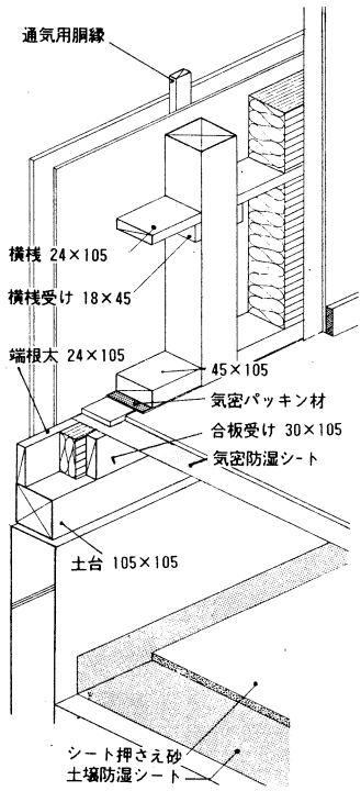
図一七 外壁下部 (横棧構法・プラットフォーム構法)
