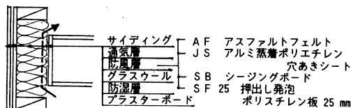
図-19 パネル概要図
