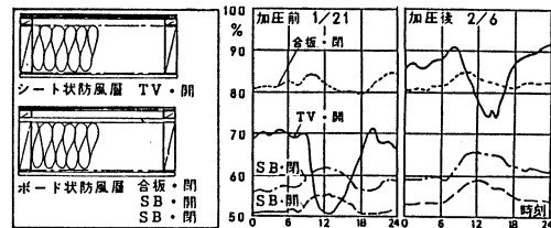
図-34 通気層壁
