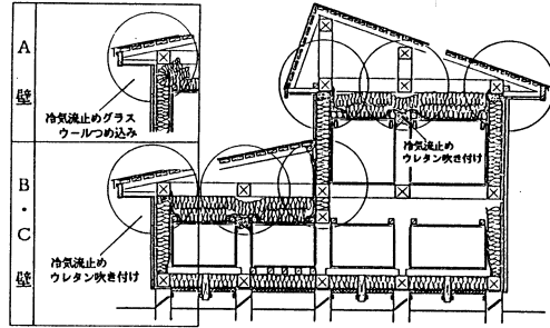
図-46 改修概要図(各取り合い部)
