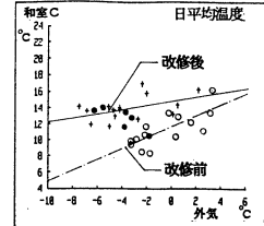
図-50 外気-2階和室C
