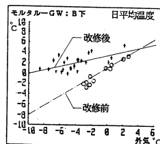
図-56 外気-B壁内温度(下)
