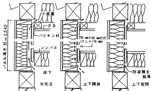
図-12 モデル壁の設定
