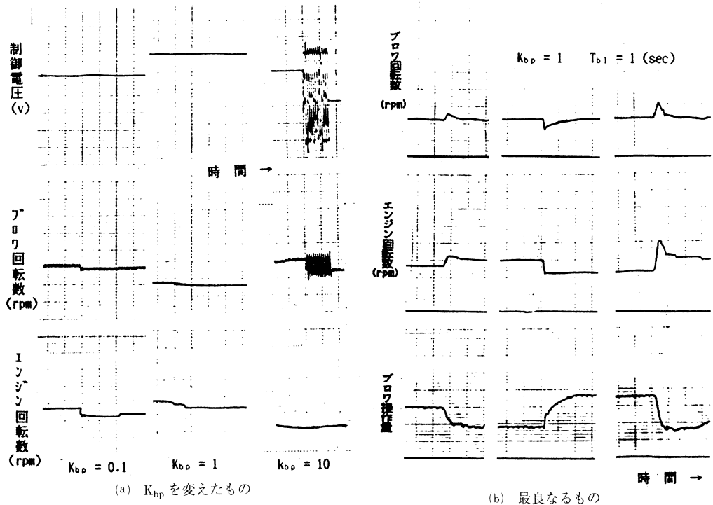
図—4 プロア回転速度制御実験
