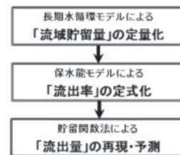
図9 流域貯留量を助案した洪水流出計算のフロー
