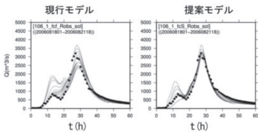
図 12 洪水予測計算の結果（モデルは一般化貯留関数法+カルマンフィルタ、予測雨量は実測雨量を使用 ●は実測流量、実線は LT 12 時間までの予測流量の結果） (沙流川水系・二風谷ダム 2006/8/18～8/21)
