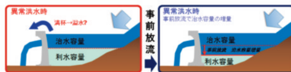
図6 異常な洪水に備えた「事前放流」のイメージ
