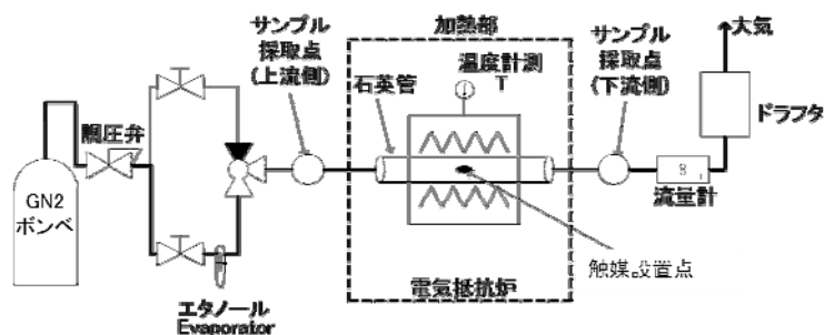
図1 実験装置概要
