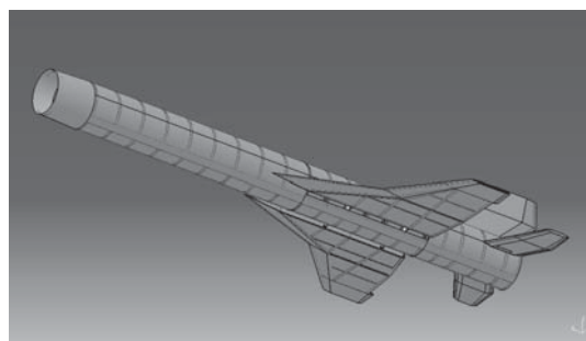
Fig. 4.9 機体全体構造図(翼胴ファイレット、エンジン、インテークコーン除く)
