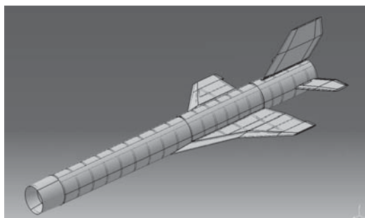
Fig. 4.9 機体全体構造図(翼胴ファイレット、エンジン、インテークコーン除く)
