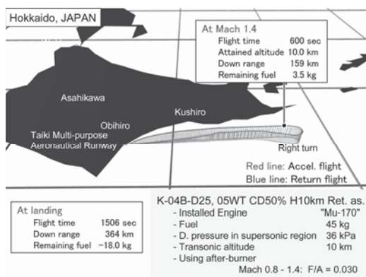
(a) 飛行経路の鳥瞰図.
