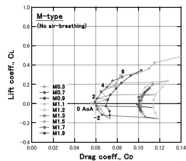
M 型機体形状 ・主翼前縁後退角 45 deg.(ストレイク部: 70 deg.) ・ Re = 1.2 - 3.1 \times 10^7 / m ・エンジン内部の空気吸い込み模擬: なし
