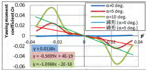
Fig. 3.2. C_n vs. \dot{p} .
