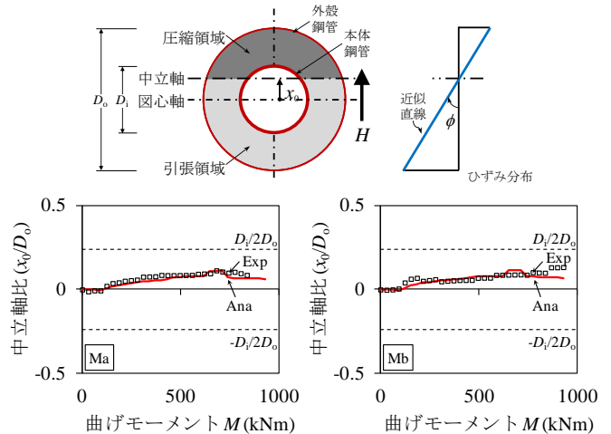
図12 M- x_0/D_0 関係 ( z=0.3\text{m} )
