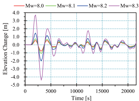
図-4 各 M_w に対する新釧路川河口における水位変動
