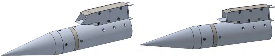
図1 インテーク風洞試験供試体モデル 左：オリジナル側壁形状モデル 右：45°垂直側壁形状モデル
